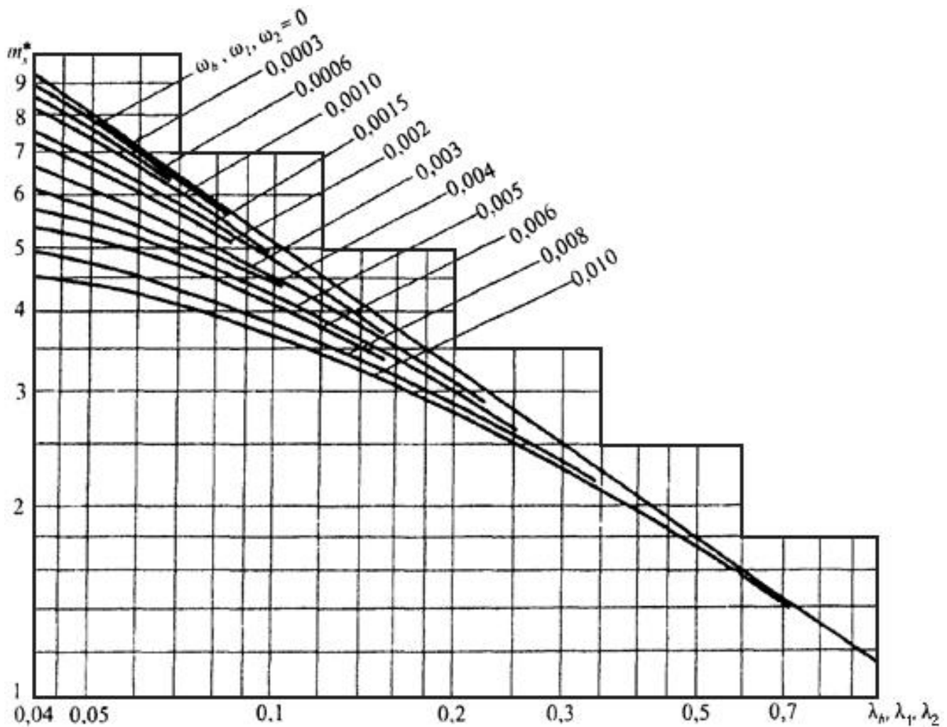
Рисунок 2 - График для определения значений коэффициента интенсификации напряжений
