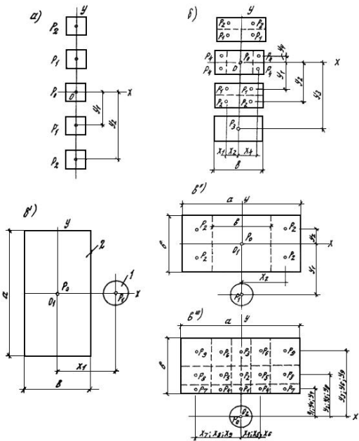
а - нечетное число одинаковых нагрузок, расположенных в один ряд; б - то же, при четном
