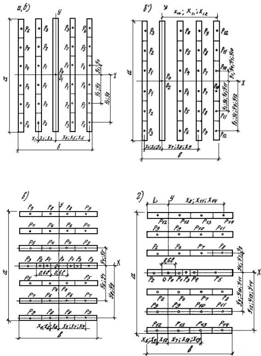
а, в - нагрузки, равномерно распределенные по длине параллельных следов (от прокладок под тяжелые предметы, от штабелей цилиндрических валов и др.) при b \leq 4,4l ; а > b; б, в' - то же, при b > 4,4l ; а > b
